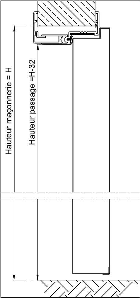
Coupe B-B' - Echelle 1/4
