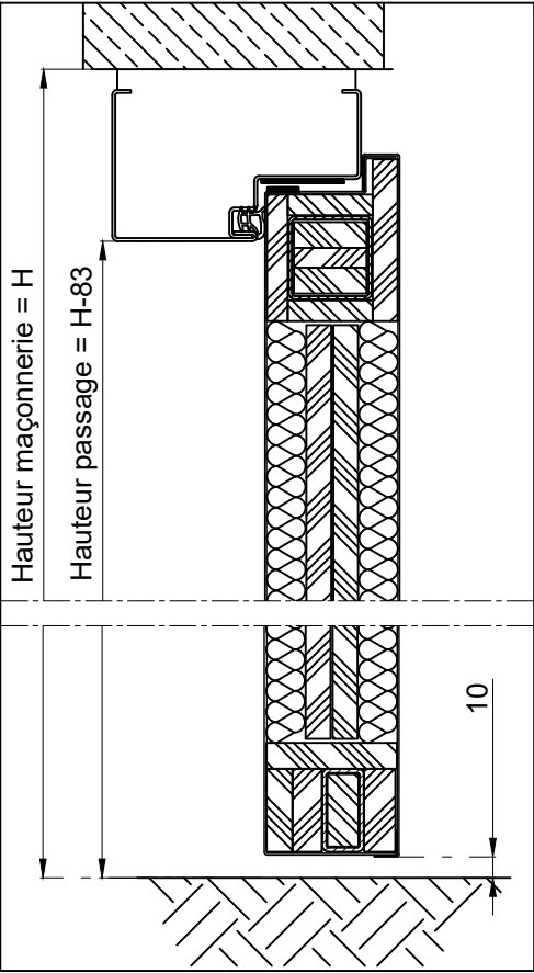
Coupe B-B' - Echelle 1/4
