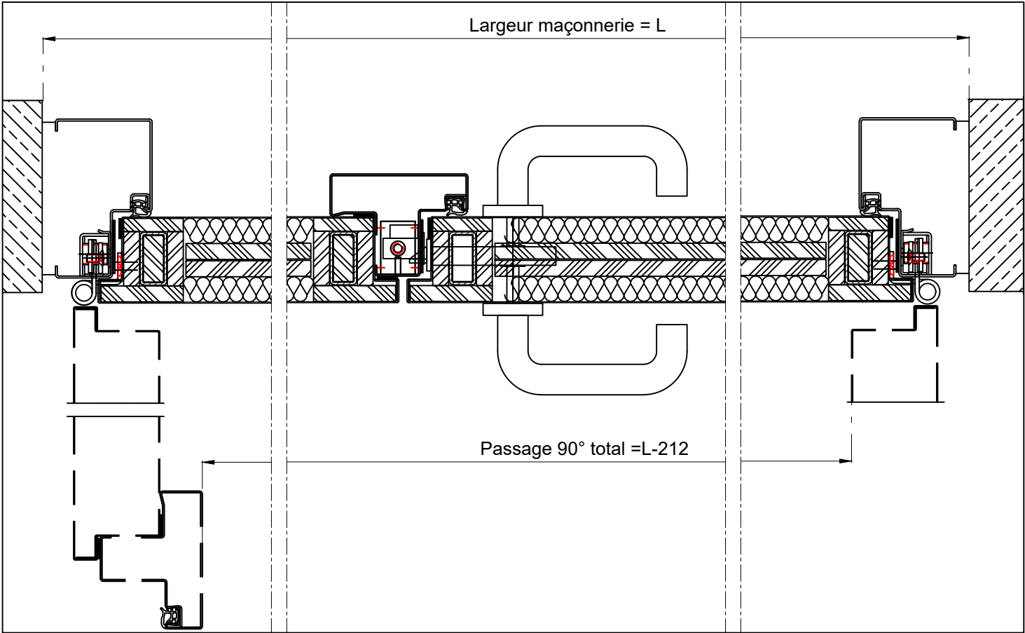
Coupe A-A' - Echelle 1/4
