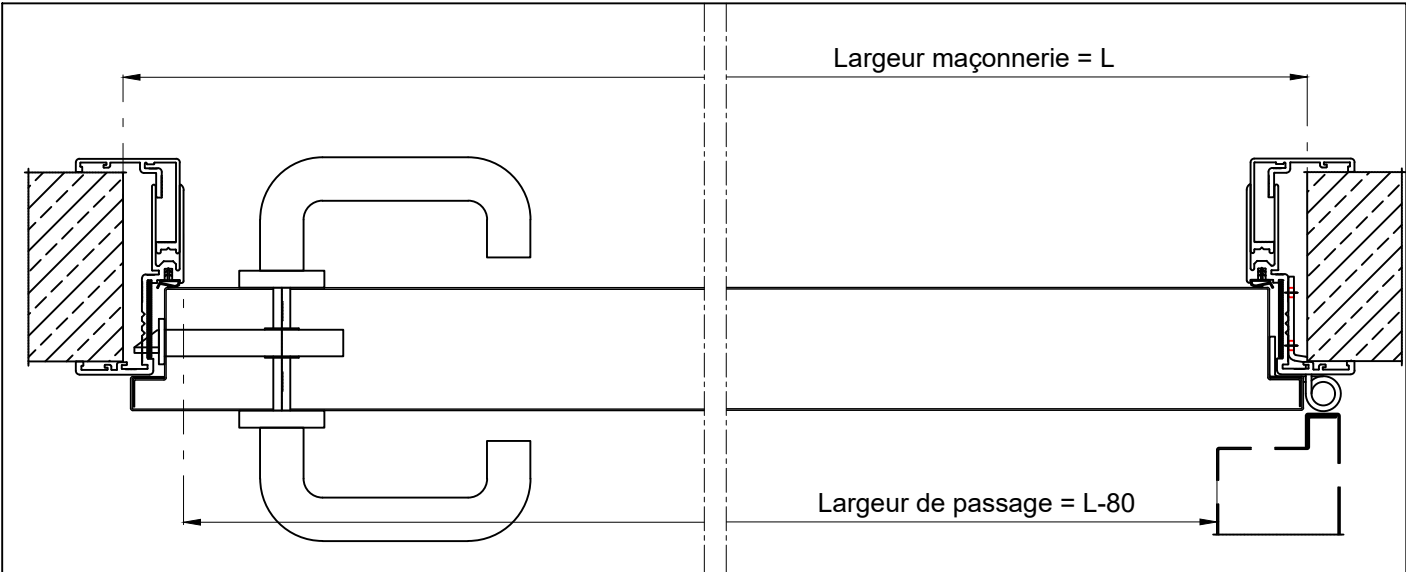
Coupe A-A' - Echelle 1/4
