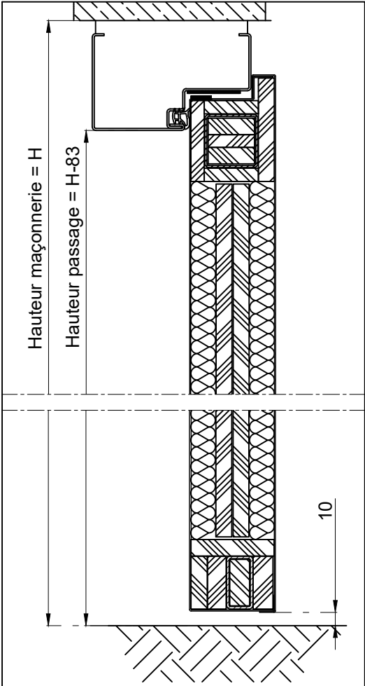
Coupe B-B' - Echelle 1/4
