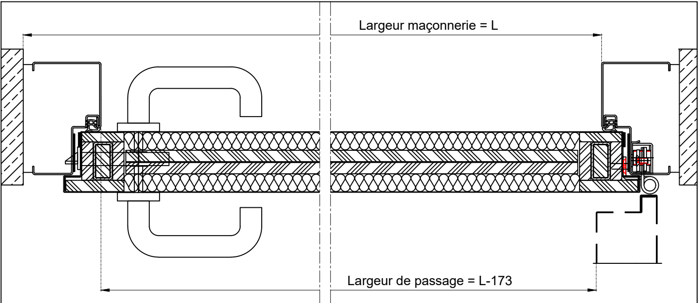
Coupe A-A' - Echelle 1/4
