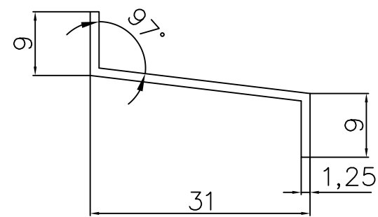
Rejet d'eau 2:1
