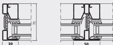
Cadre / vitrage fixe
