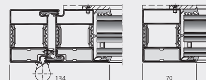
Portes pare-balles FB4
